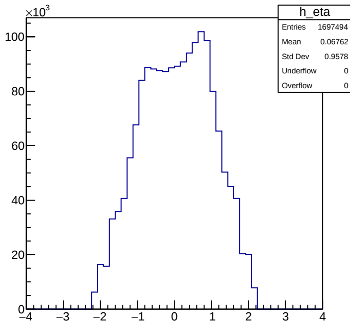
eta Process 3
