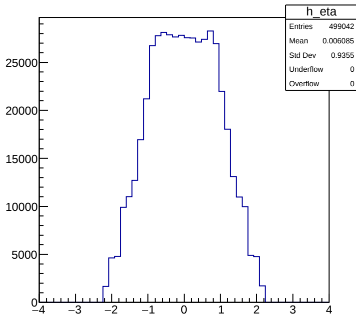
eta Process 4
