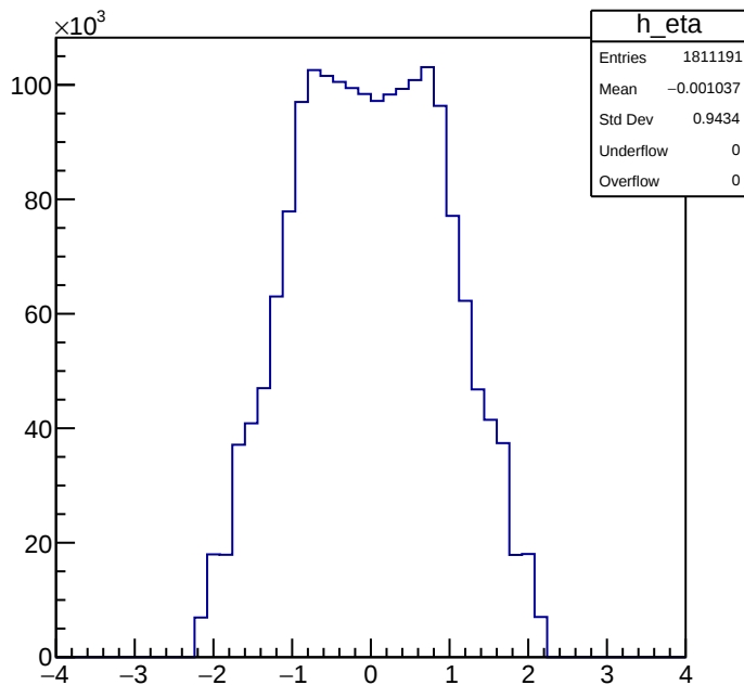
eta Process 1
