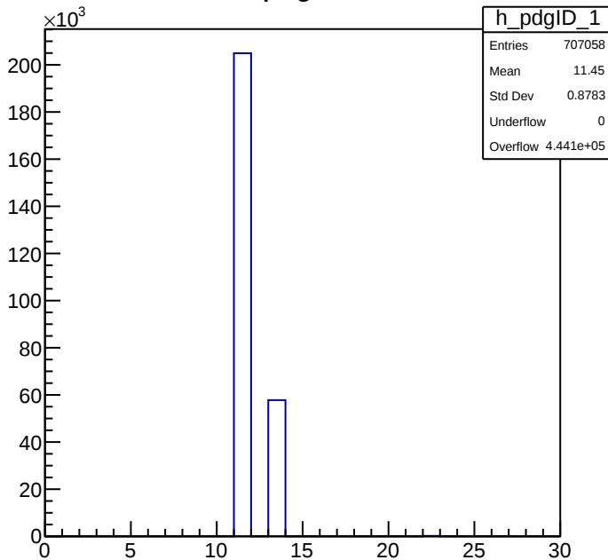
pdgID
