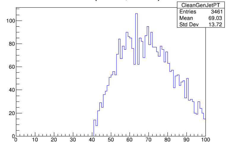
Clean PT {GenJet1, GenJet2}
