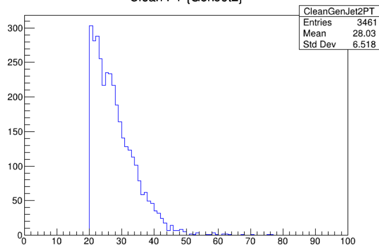
Clean PT {GenJet2}
