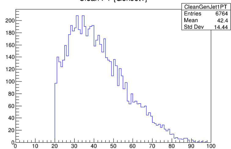
Clean PT {GenJet1}
