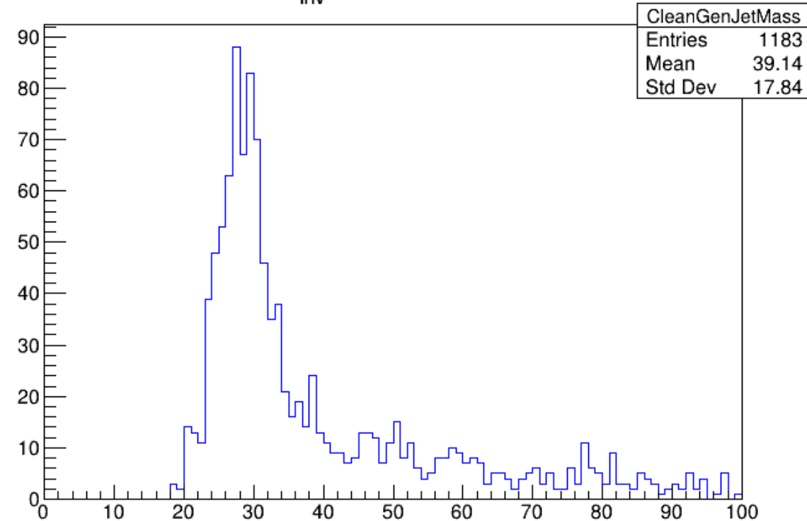
Clean M_{inv} {GenJet1, GenJet2}
