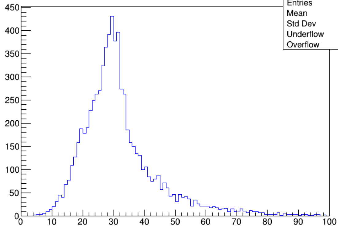
M_{inv} {GenJet}
