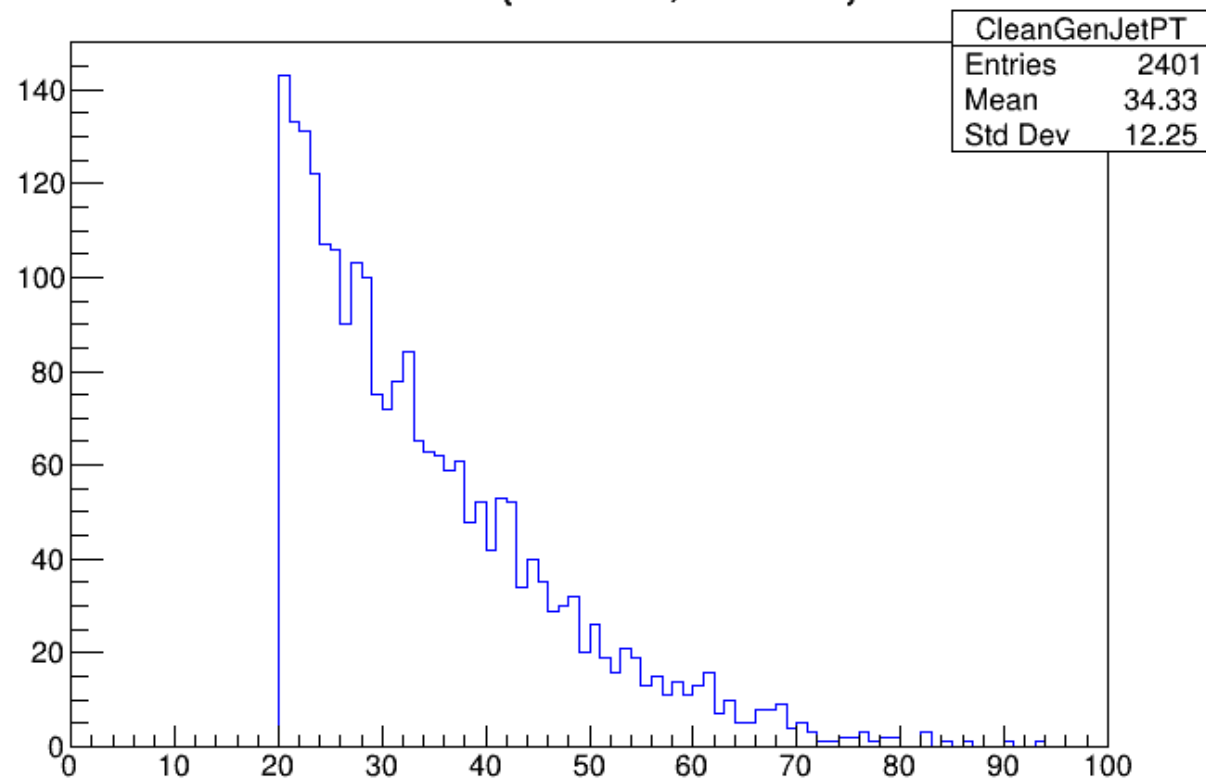
Clean PT {GenJet1, GenJet2}
