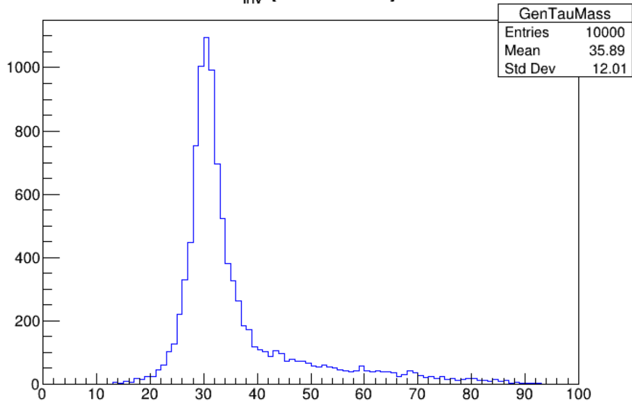
M_{\text{inv}} {GenTau all}
