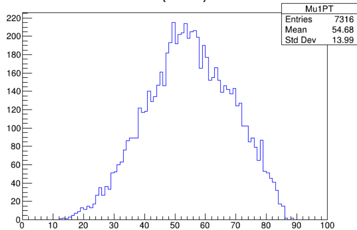
PT {Muon1}
