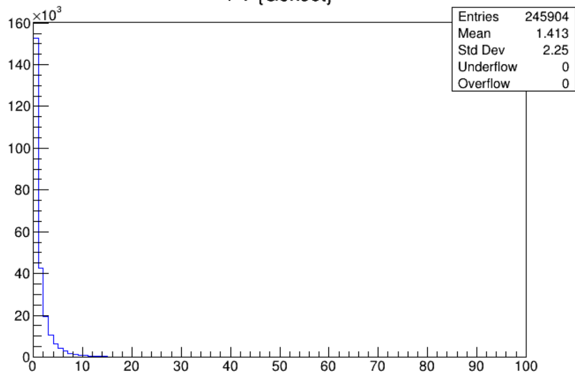
PT {GenJet}
