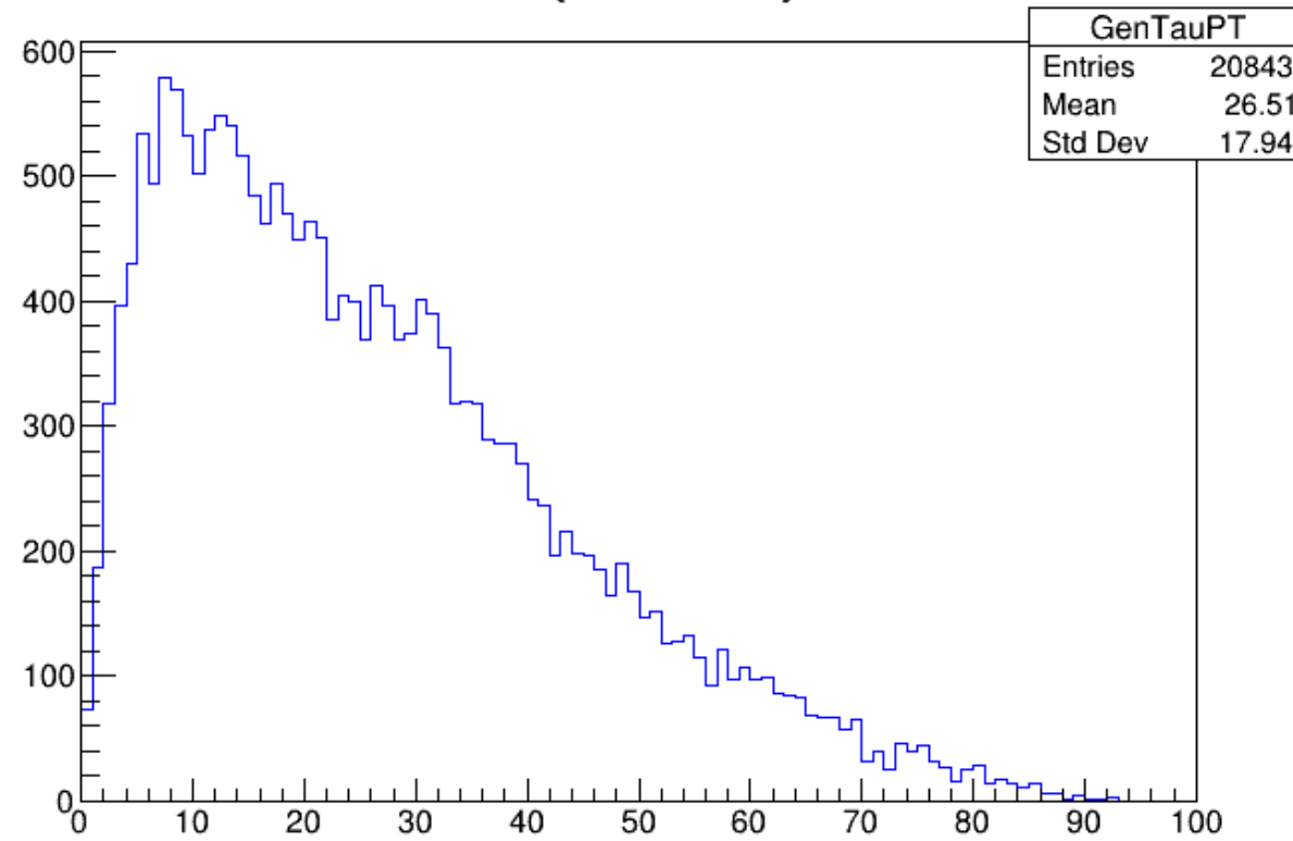
PT {GenTau all}
