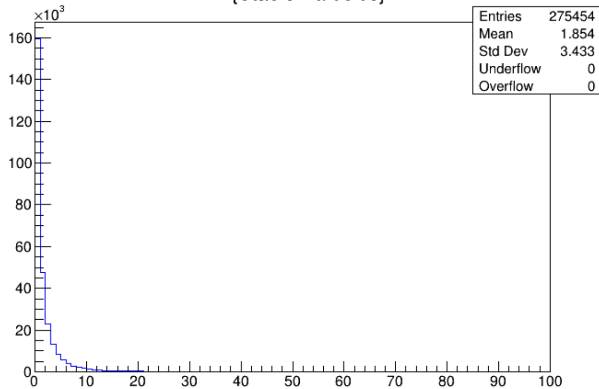
PT {Stable Particles}
