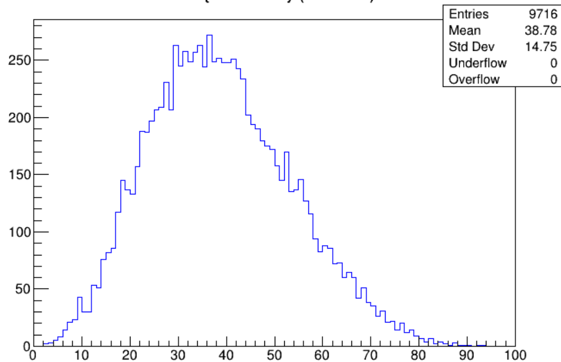
PT {RecTau1} (ZBoson)
