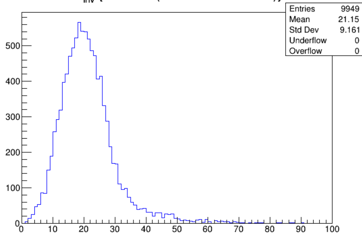
M_{\text{inv}} {a Boson (VisTau1 + VisTau2)}
