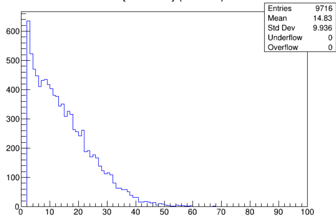
PT {RecTau2} (ZBoson)
