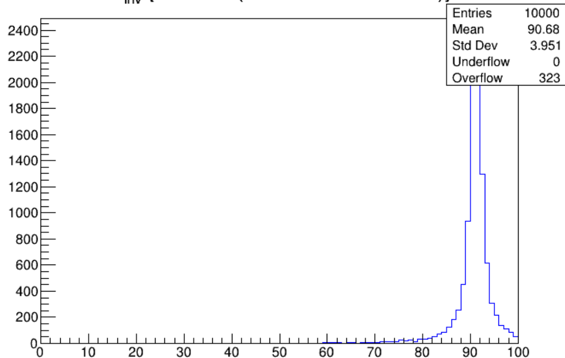
M_{inv} {Z Boson (GenTau1 + GenTau2)}
